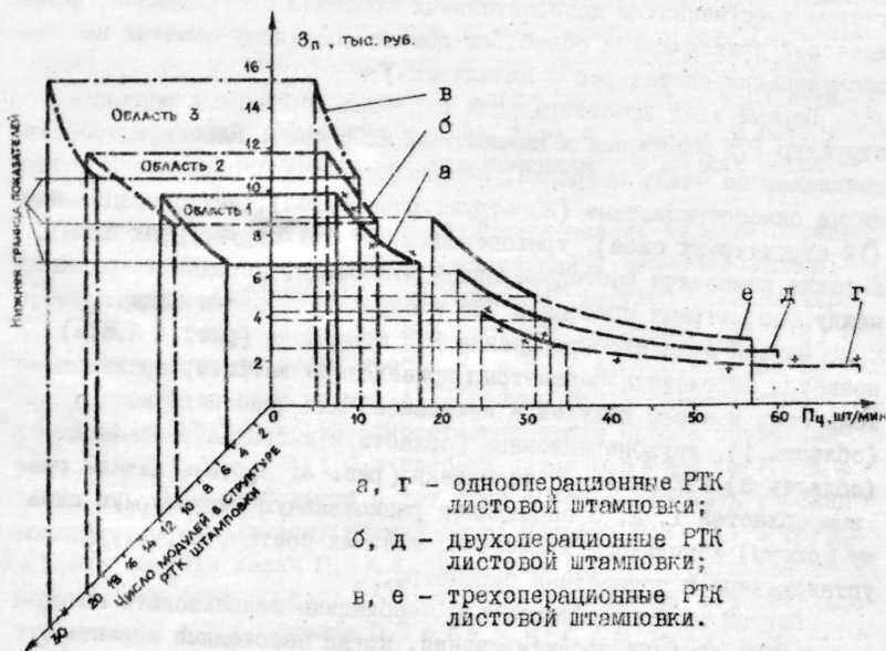
Рис. 4. Показатели эффективности РТК листовой штамповки : а, б, в - 1-й этап проектирования; г, д, е - II-ой этап проектирования
