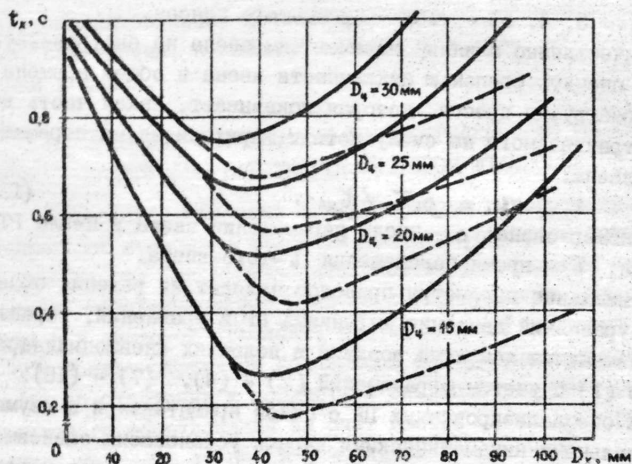
Рис. 3. Влияние конструктивных параметров приводов специализированных ПР на его быстродействие
