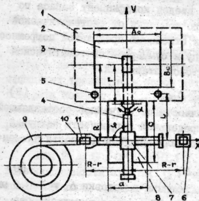
Рис. 2. Схема, поясняющая компоновку РТК листовой штамповки мелких деталей
