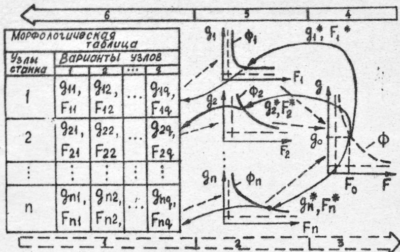
Рис. 2. Последовательность двухуровневой оптимизации конструкции станочных узлов.
