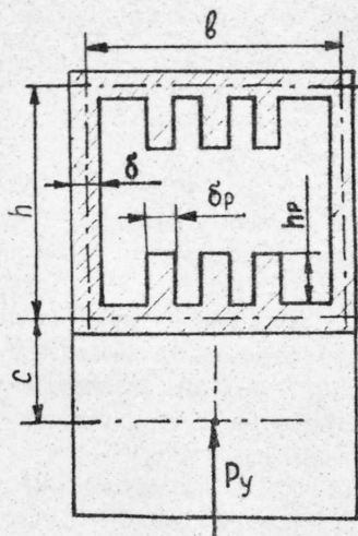
Рис. 4. Расчетная схема сечения стойки станка.
