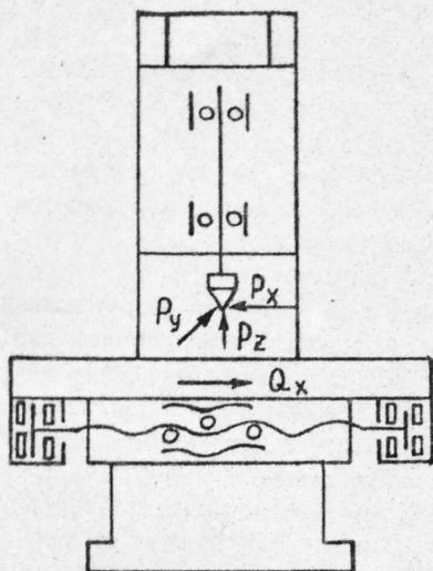
Рис. 3. Схема пространственного нагружения ИС станка.
