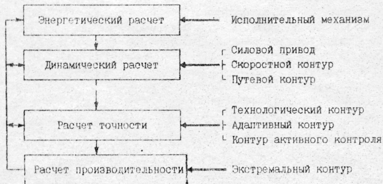
Рис. 5. Последовательность проектирования системы ЧПУ станка.
