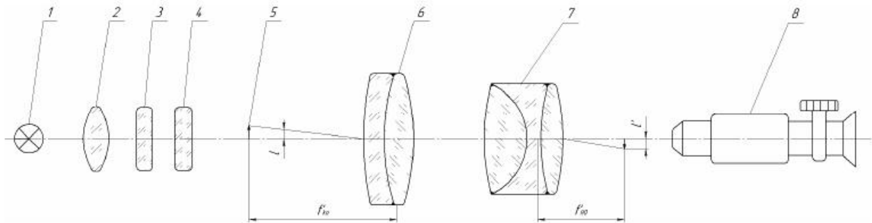
Рис. 1. Схема установки для измерения по методу увеличения:
