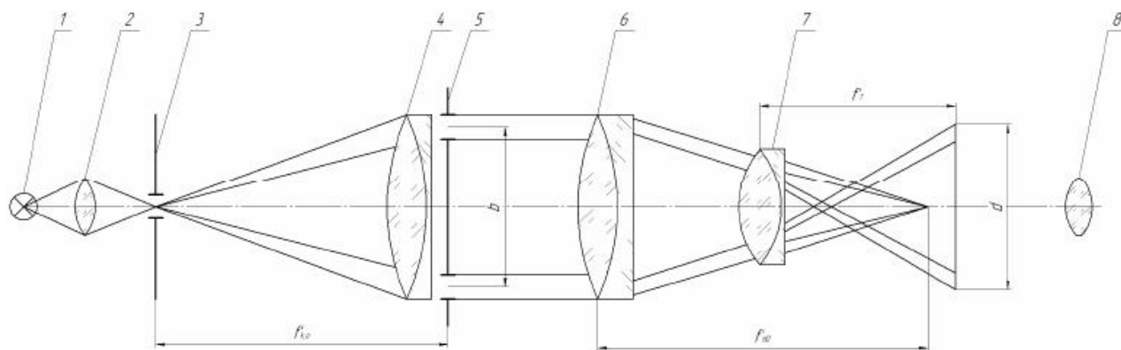
Рис. 2. Схема установки для измерения по методу Фабри — Юдина:
