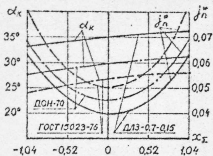
Рис. 1. Изменение угла давления \alpha_{\kappa} и бокового зазора j_n^*
