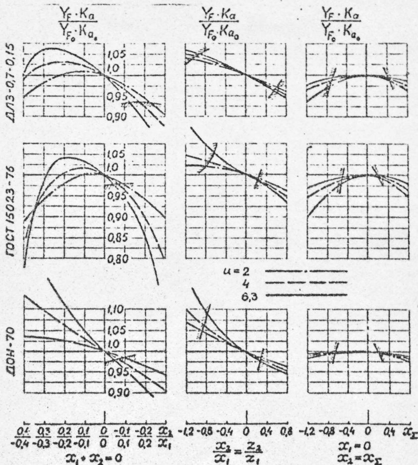
Рис. 8. Изменение изгибной прочности ненулевых передач Новикова ДЛЗ относительно нулевой передачи
