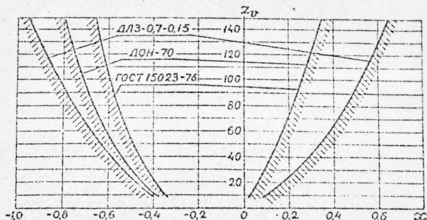
Рис.5. Рекомендуемые блокирующие контуры выбора коэффициентов смещений X
