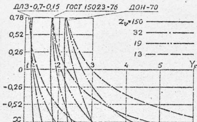
Рис.6. Изменение коэффициента формы зуба Y_F
