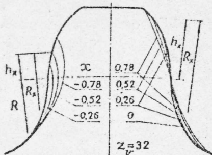
Рис. 4. Характер подреза головки зуба
