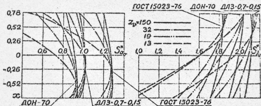
Рис. 3. Изменение толщины головки S_{a_v}^* и ножки S_{f_v}^* зуба по хорде, проходящей через номинальную точку контакта
