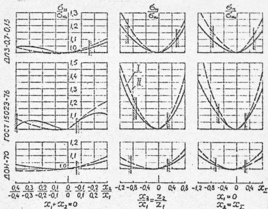
Рис.7. Относительное изменение максимальных контактных напряжений \sigma_H в зацепной - I и доцепной - II зонах контакта ненулевых передач Новикова ДЛЗ с числами зубьев z_2/z_1 = 77/19
