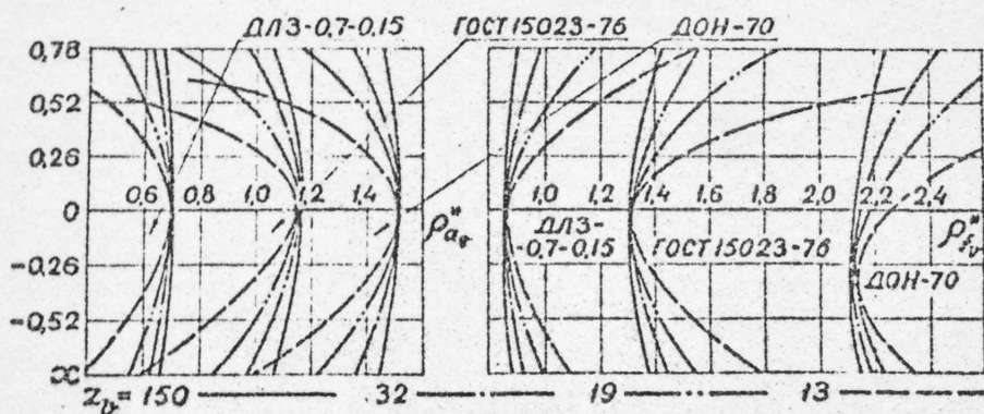
Рис. 2. Изменение радиусов кривизны профилей головки \rho_{a_v}^* и ножки \rho_{f_v}^* зуба в номинальной точке контакта
