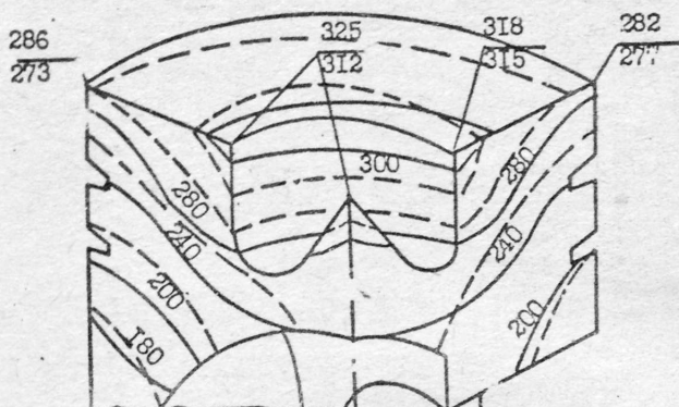
Рис.3.Трёхмерное температурное поле поршня \varnothing 120 мм. Числитель и (—) без охлаждения; знаменатель и (---) со струйным охлаждением.
