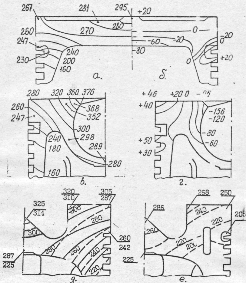
Рис.2. Расчетно-экспериментальные поля температур и окружающих термических напряжений поршней дизелей ГЧН 7,6/8,0 (а), ГЧН II/II,5 (б), 8ЧН I3/I4 (д,е) без охлаждения (в), при организации струйных (а, в) и полостных (е) способов охлаждения на номинальном режиме работы дизеля.
