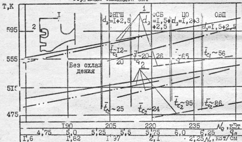
Рис.4. Сравнительная характеристика эффективности различных способов масляного охлаждения поршней дизеля 6ЧН 13/14. ФВГШ—форсунка на верхней головке шатуна; ФСБ—форсунка на стенке блока; ЦО—циркуляционное охлаждение; ОВП—охлаждение взбалтыванием масла в частично-заполненной полости; d_3 —эквивалентный диаметр соплового отверстия форсунки (мм); \bar{t}_1 и \bar{t}_2 —удельные относительные снижения температур 1-го и 2-го участков поршня (К.кВт.ч/л); — максимальные температуры неохлаждаемых поршней; охлаждаемых: --- ФВГШ, -.- ФСБ, .-. ЦО и ОВП; N_p —поршневая мощность; q_n —критерий тепловой напряженности поршней Л.К.Костина.
