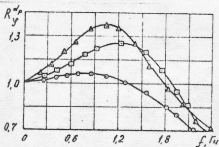
Рис.1. Экспериментальные АЧХ САР частоты вращения дизеля КАМАЗ-740.
