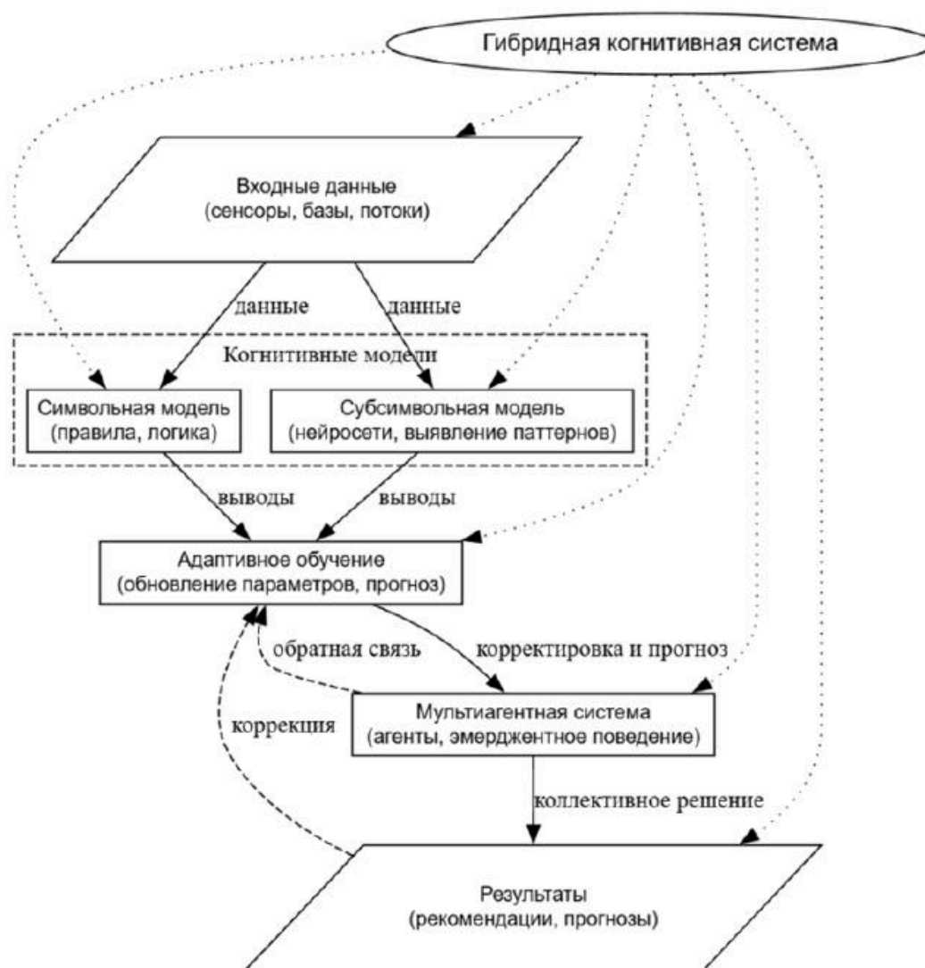
Структура гибридной когнитивной системы и потоки данных
